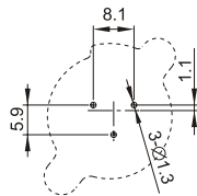
P.C.B LAYDUT ±0.1 BOTTOM VIEW
